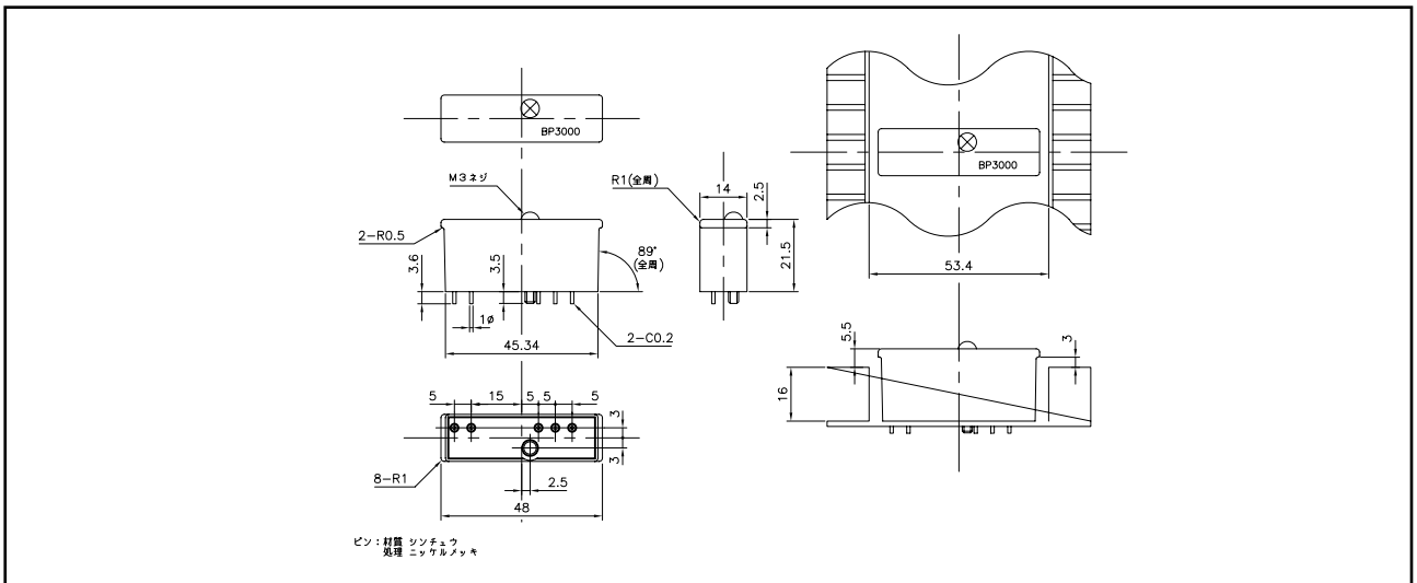
BP3000 ソケットカバー
