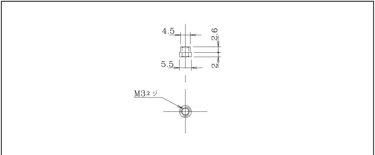
M3500-TB-BOSS モジュール固定用ナット
