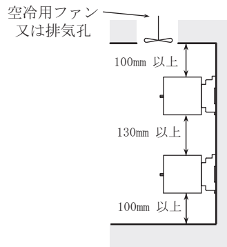
設置例
