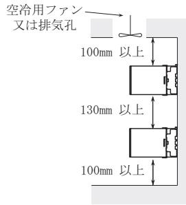
設置例
