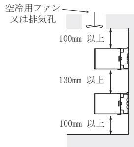
設置例
